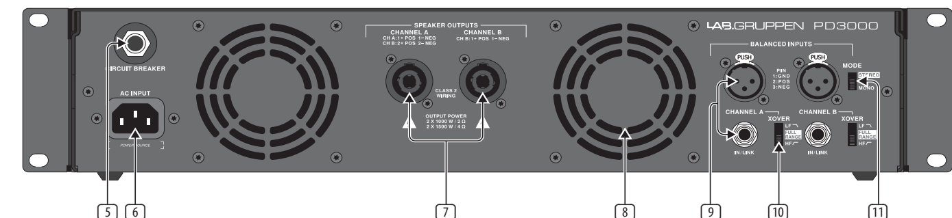
Fig. 2: Pannello posteriore del PD3000
